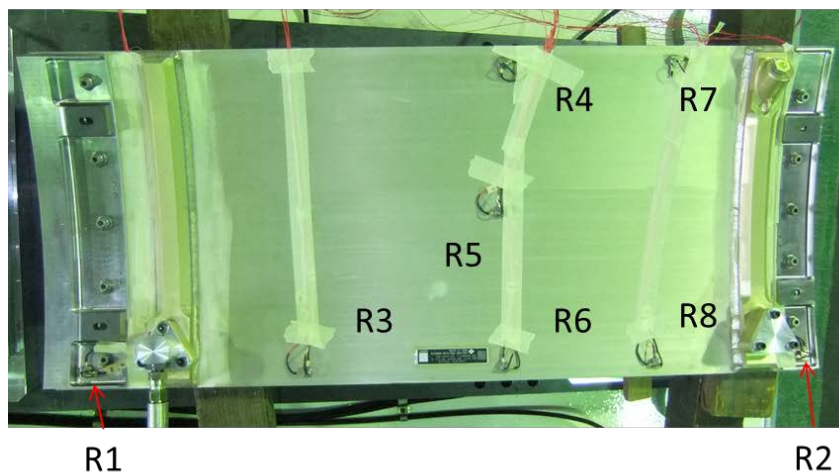
R1 ～ R8 3軸加速度計と位置
