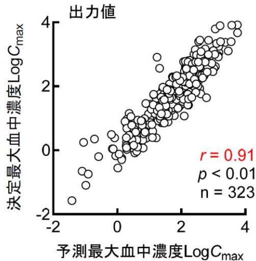
図 9 血中濃度の実測値と予測値
