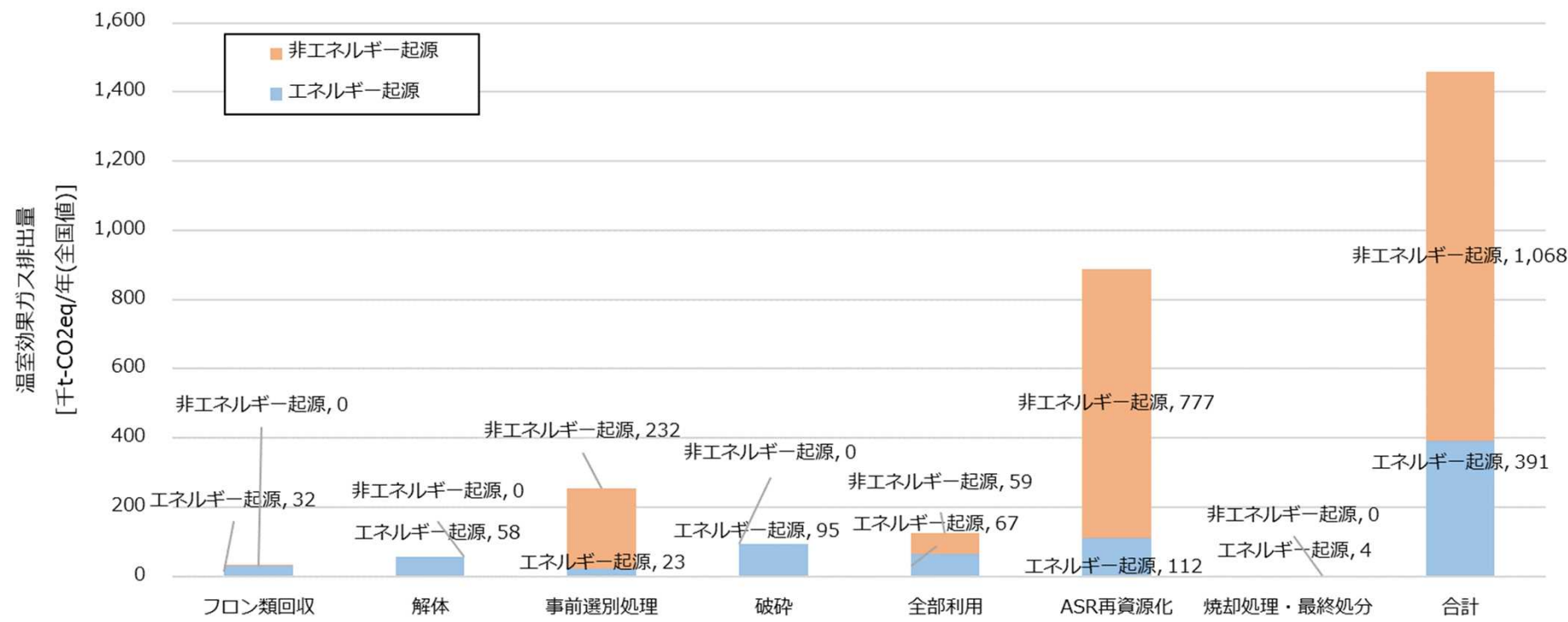
【自動車リサイクルにおける温室効果ガス排出量の試算結果】
