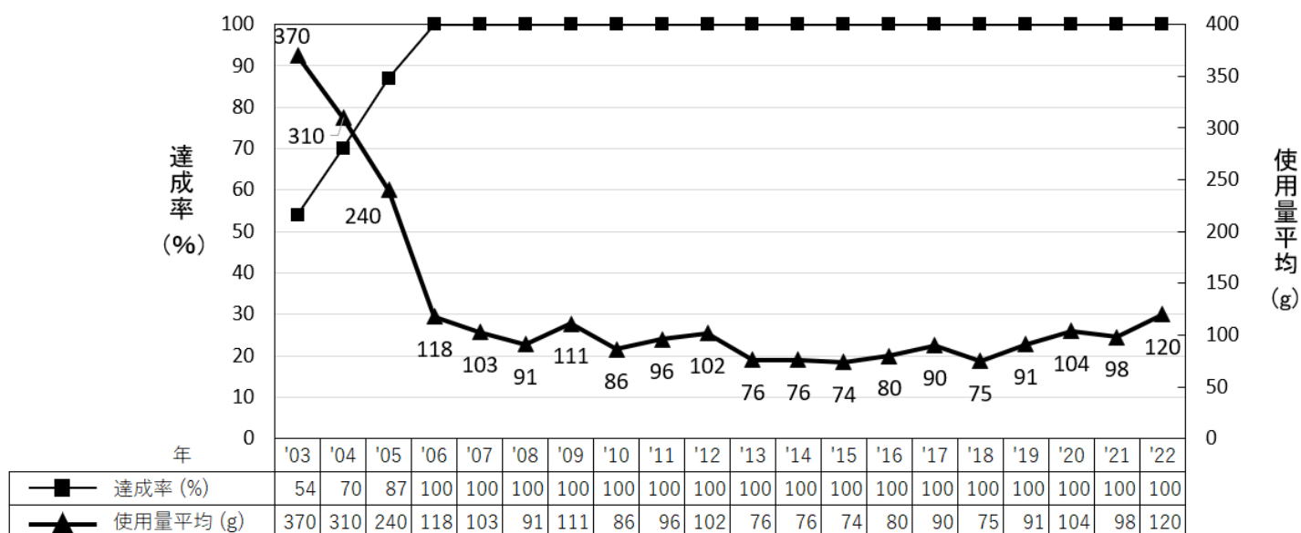
図1. 鉛使用量削減状況(乗用車平均)2003年～2022年(1～12月)推移
