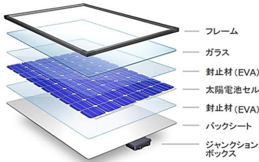
シリコン電池の構造（出所：NEDO）
