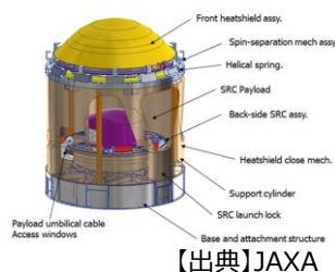
【出典】JAXA 構想中の彗星からの サンプル回収カプセル
