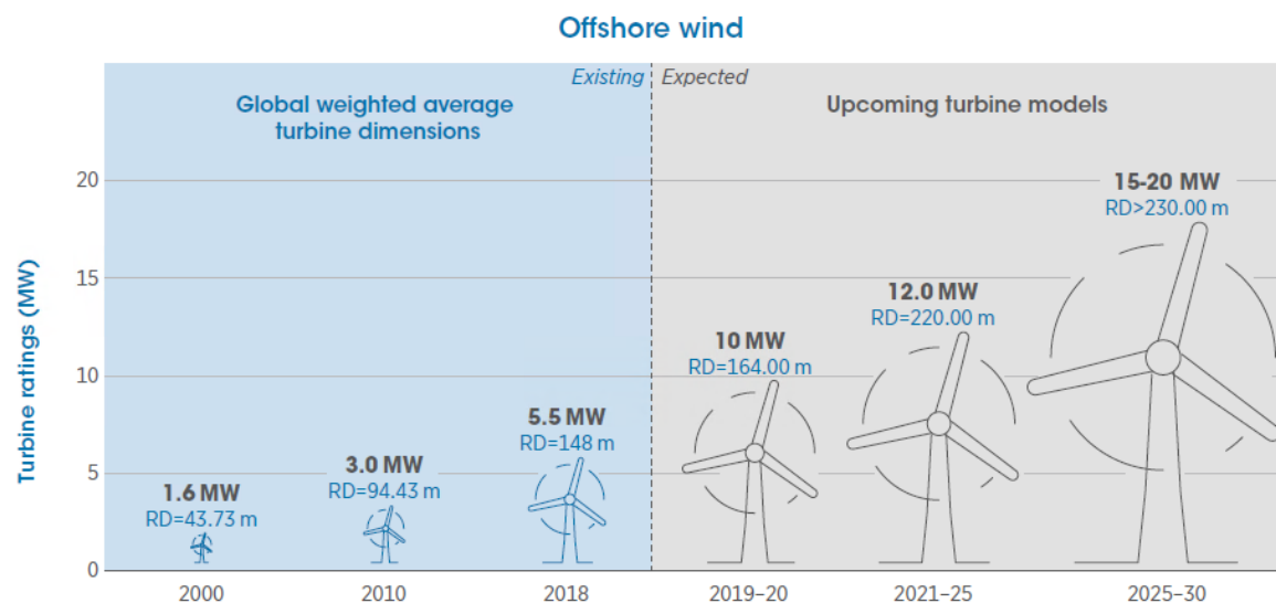
＜着床式洋上風力発電設備の風車規模の推移＞
