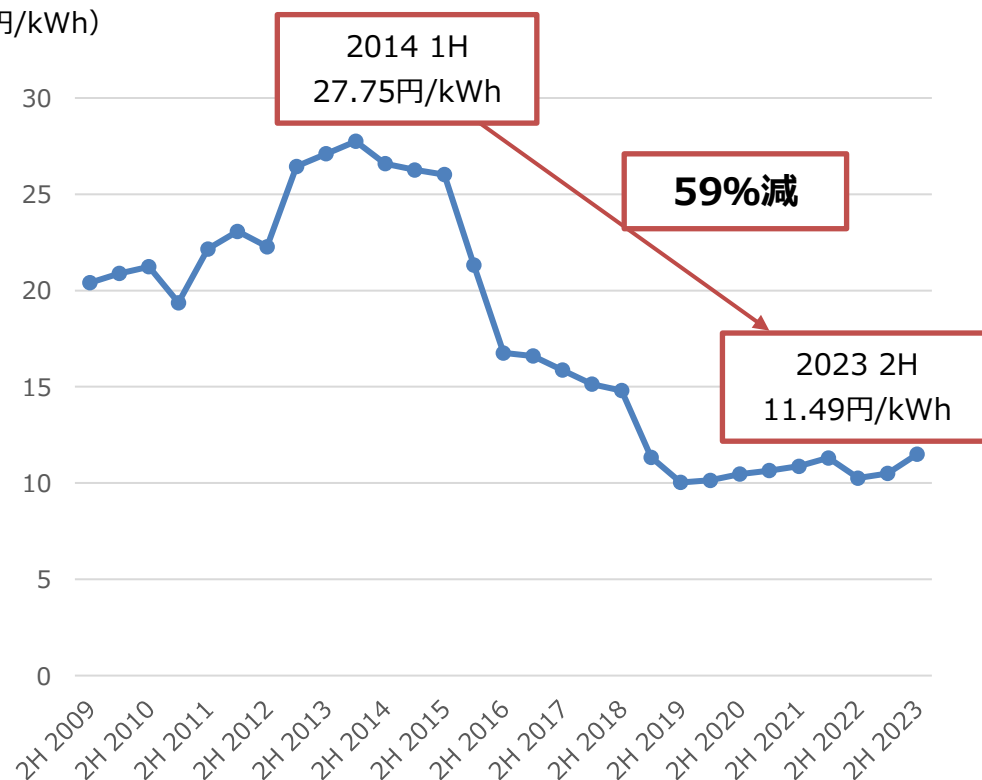
＜世界における洋上風力発電のLCOEの推移＞
