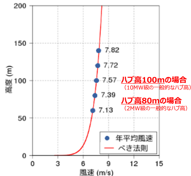
＜風速の鉛直分布＞
