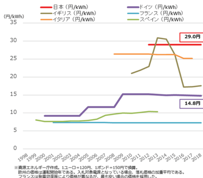
【参考 53】 中小水力発電（200kW）の各国の価格
