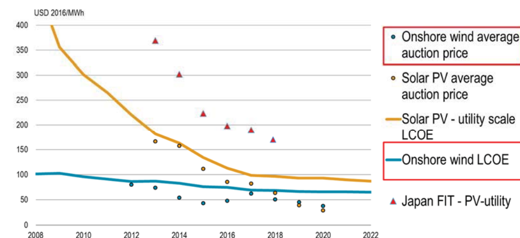
【参考 35】 陸上風力発電の世界のコスト動向
