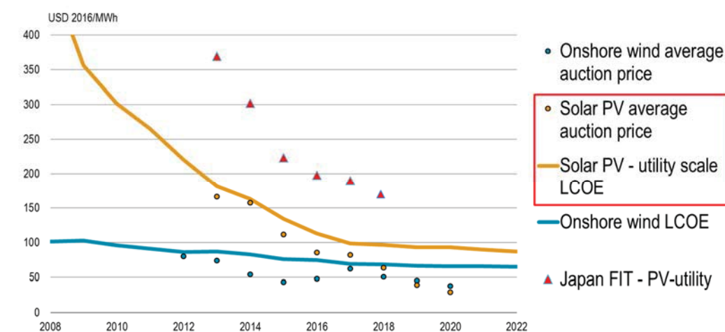
【参考4】世界の事業用太陽光発電のコスト動向
