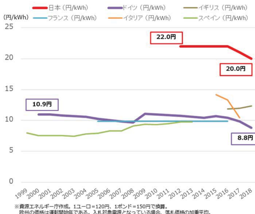
【参考 34】 風力発電(陸上、20,000kW)の各国の価格
