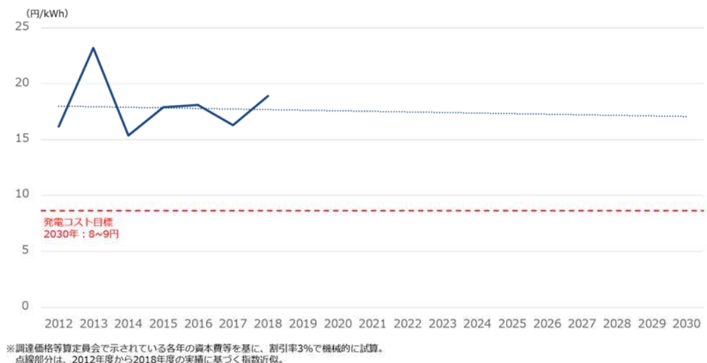
【参考 37】日本の陸上風力発電のコスト動向（実績）
