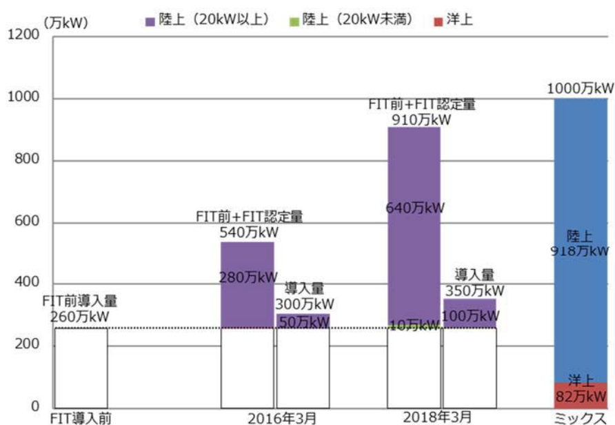
【参考 33】 風力発電の FIT 認定量と導入量
