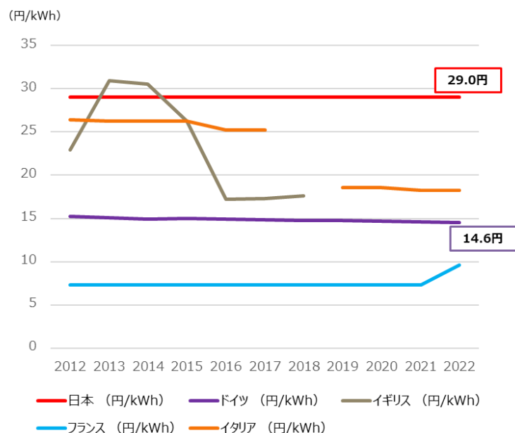
【参考 63】 中小水力発電（200kW）の各国の価格
