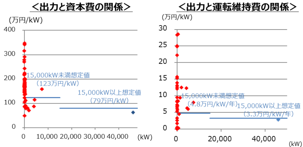
【参考 55】地熱発電の出力と資本費・運転維持費の関係
