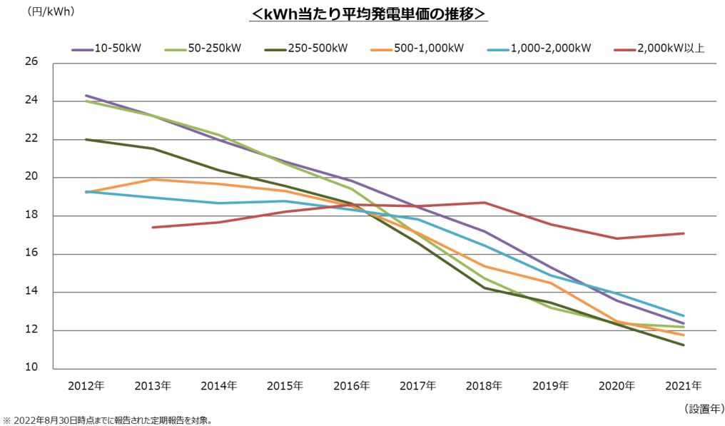
【参考 15】事業用太陽光発電の設置年別の kWh 当たり発電コスト
