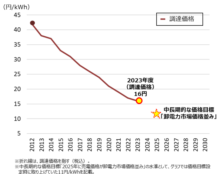
【参考 33】住宅用太陽光発電の現行の価格目標と調達価格の推移
