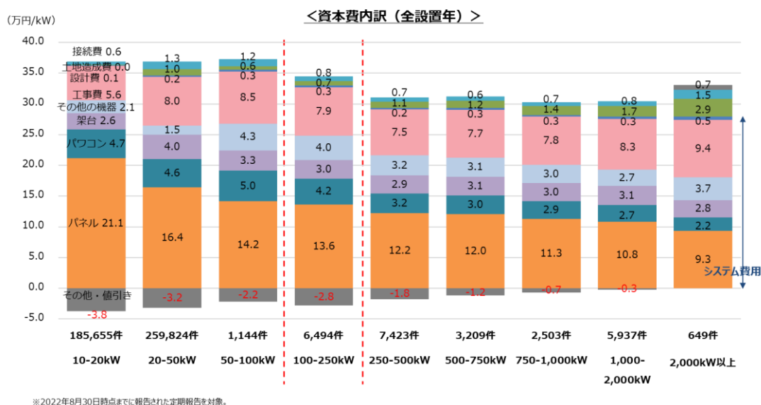
【参考 93】事業用太陽光発電の資本費及びその構成（規模別）
