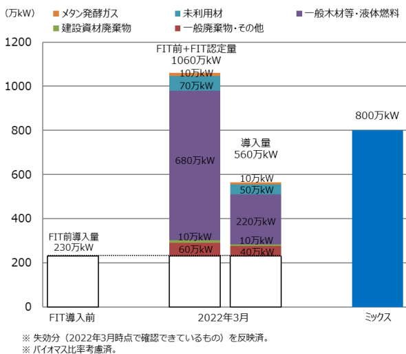
【参考 73】 バイオマス発電の FIT 認定量
