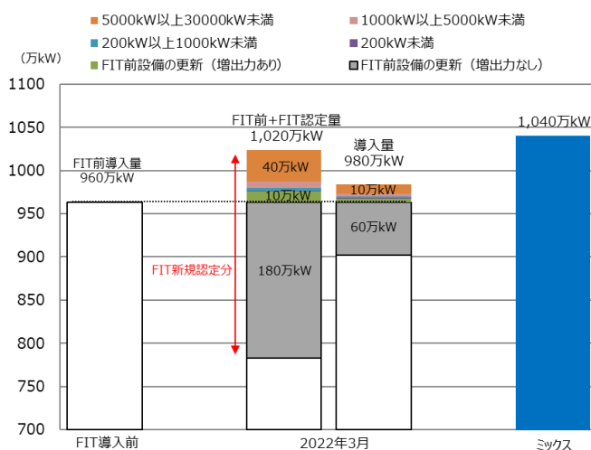
【参考 60】 中小水力発電の FIT・FIP 認定量・導入量
