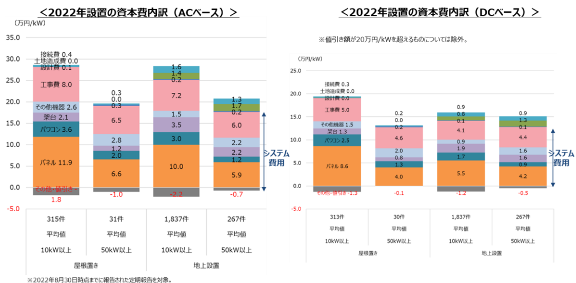
【参考19】2022年設置の事業用太陽光の資本費内訳の詳細
