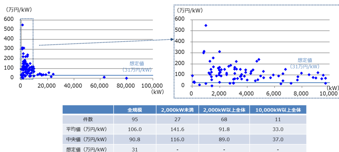
【参考 84】一般廃棄物その他バイオマス発電の資本費
