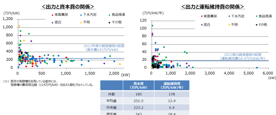
【参考 87】メタン発酵バイオガス発電の資本費・運転維持費
