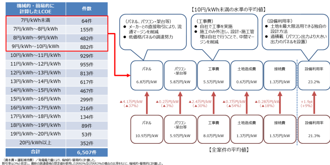
【参考 32】低コストで事業実施できている事業用太陽光発電
