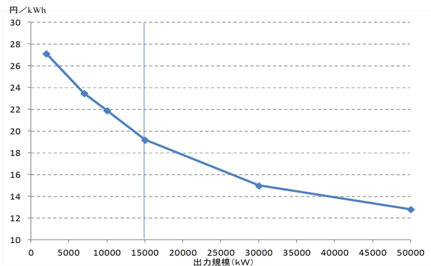
【参考5】地熱発電の出力規模別発電原価（15年平均）
