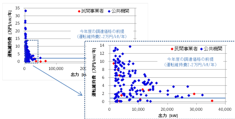
【参考 26】 廃棄物バイオマス発電の出力と運転維持費の関係
