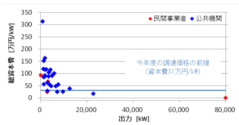
【参考 25】 廃棄物バイオマス発電の出力と資本費の関係
