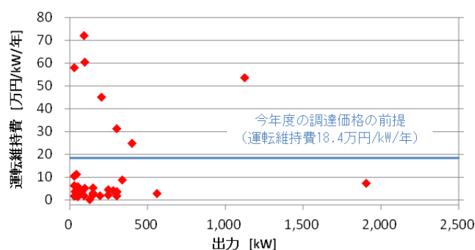
【参考 28】メタン発酵バイオガス発電の出力と実質的な運転維持費の関係
