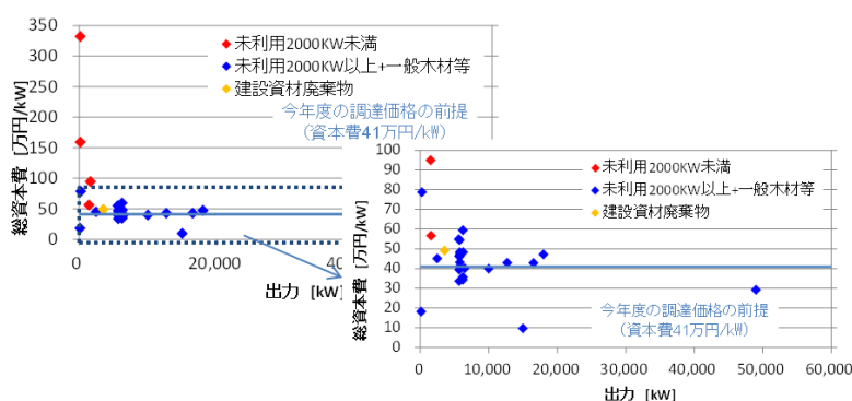
【参考 21】木質等バイオマス発電の出力と資本費の関係
