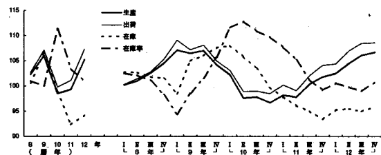
第1図 鋳工業生産・出荷・在庫・在庫率指数の推移 (平成7年=100、季節調整済)
