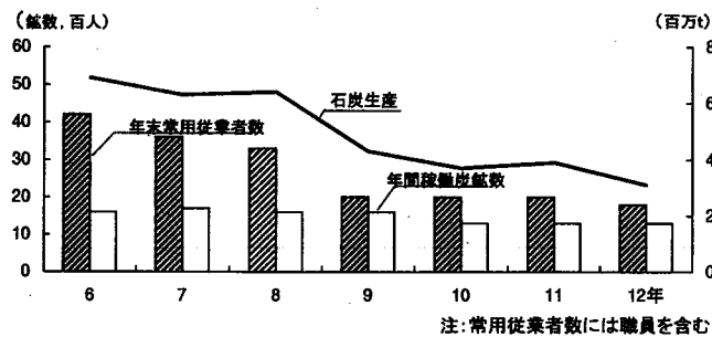
第8図 石炭生産・炭鉱数・従業者の推移
