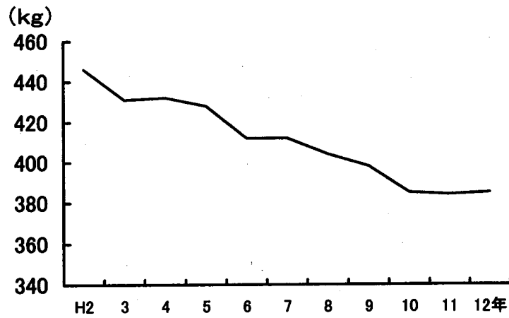
第12図 石炭コークスの消費原単位 (鉄鉄1t当たり)
