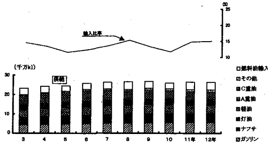
第3図 燃料油の生産・輸入及び輸入比率の推移
