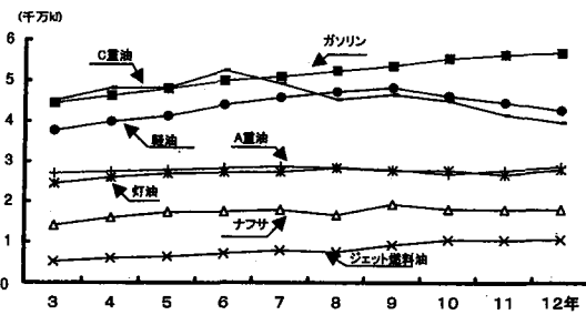
第4図 燃料油の生産推移
