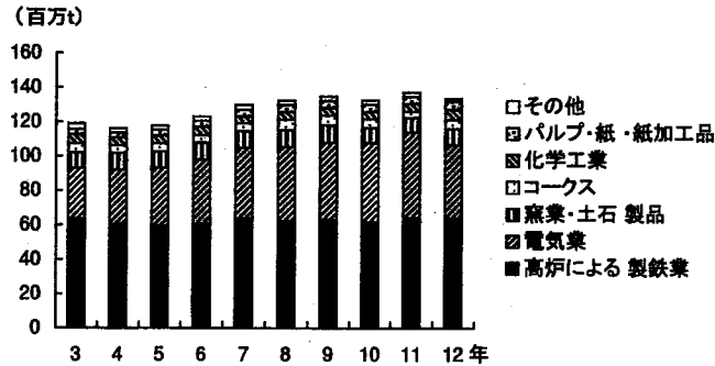
第10図 石炭の産業別販売の推移
