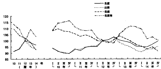
第3-1図 非鉄金属工業生産・出荷・在庫・在庫率指数の推移 (平成12年=100、季節調整済)
