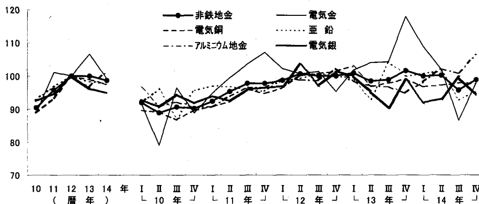
第3-4図 非鉄金属地金の生産の推移
