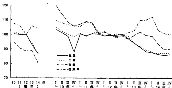
第4-1図 金属製品工業生産・出荷・在庫・在庫率 指数の推移 (平成12年=100、季節調整済)
