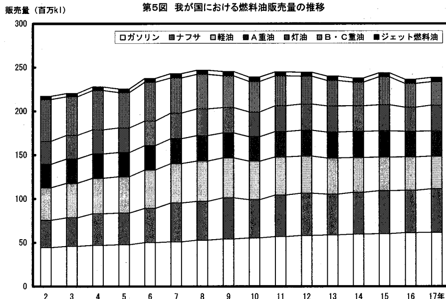
第5図 我が国における燃料油販売量の推移
