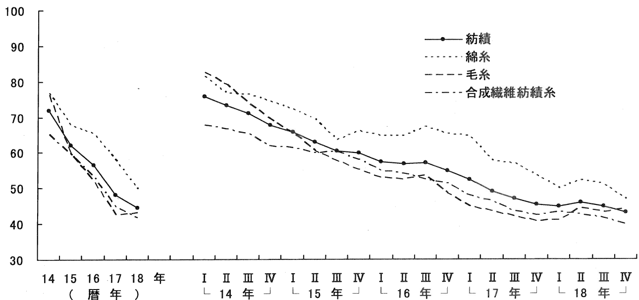
第5図 紡績の主要品目別生産の推移 (平成12年=100、季節調整済)
