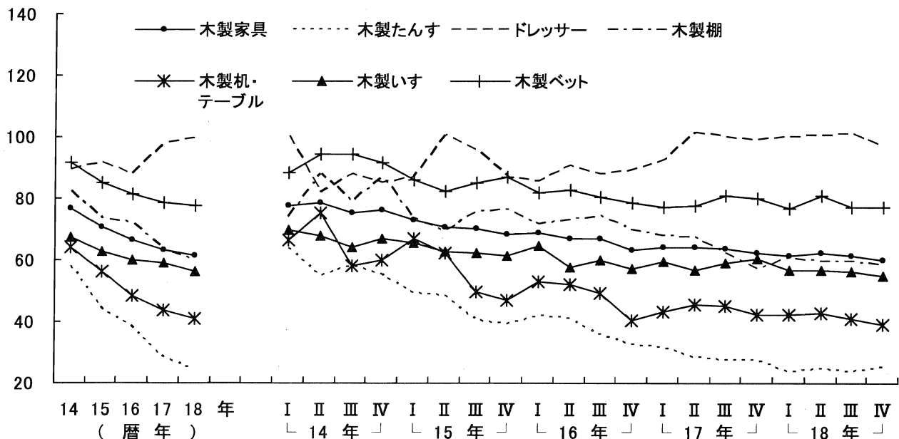
第11図 木製家具の主要品目別生産推移 (平成12年=100、季節調整済)
