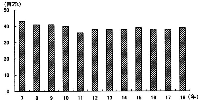
第7図 コークスの生産推移
