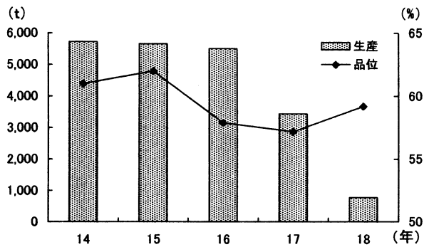
第9図 鉛(含有量)の生産量と品位
