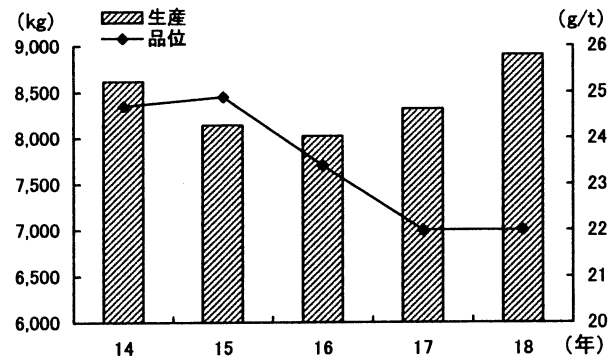
第8図 金(含有量)の生産量と品位
