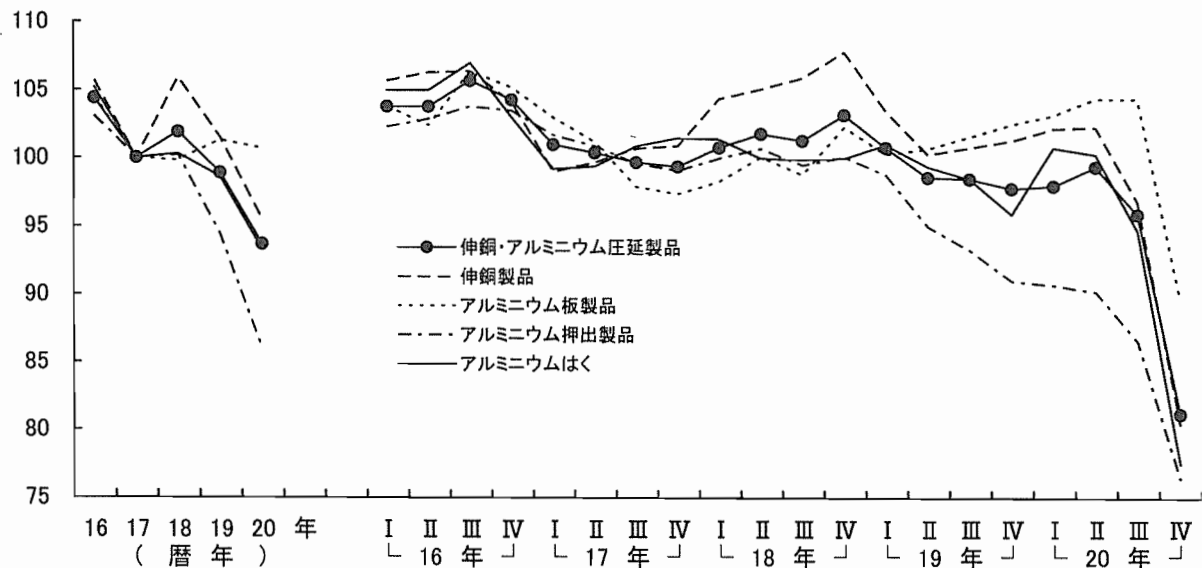
第3-4図 伸銅・アルミニウム圧延製品の生産の推移
