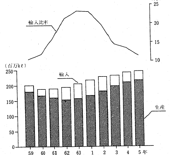
第3図 燃料油の生産、輸入及び輸入比率の推移(%)
