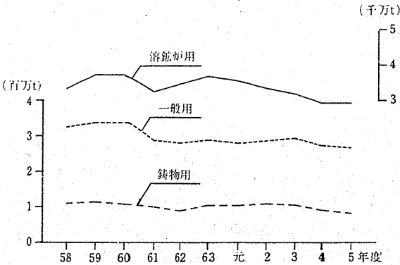
第9図 コークス品種別生産の推移
