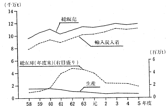
第7表 石炭総販売(輸入炭を含む) (単位：千t)
